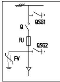
9-400 9-600 Ввод, отходящая линия
