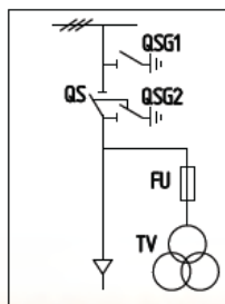
11-600ТН Трансформатор напряжения
