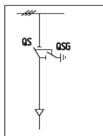
1-400 1-600 Ввод, отходящая линия
