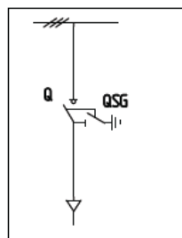
3-400 3-600 Ввод, отходящая линия
