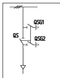
2-400 2-600 Ввод, отходящая линия
