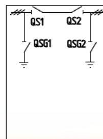
ШМП (2000, 2100, 2200, 2300, 2500, 2800, 3000 мм) Шинный мост с разъединителями
