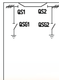
ШМР (2000, 2100, 2200, 2300, 2500, 2800, 3000мм) Шинный мост с разъединителями
