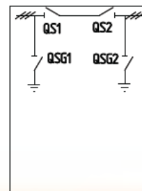
ШМР (2000, 2100, 2200, 2300, 2500, 2800, 3000 мм) Шинный мост с разъединителями
